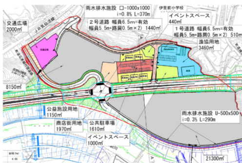
(計画図)
